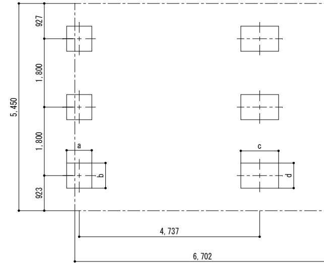
■ 基礎配置図
